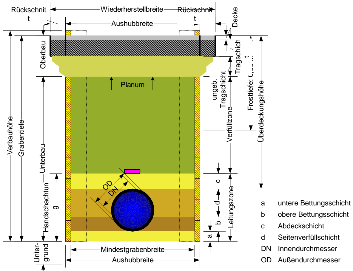
Abbildung 3 Standardgrabenprofil
