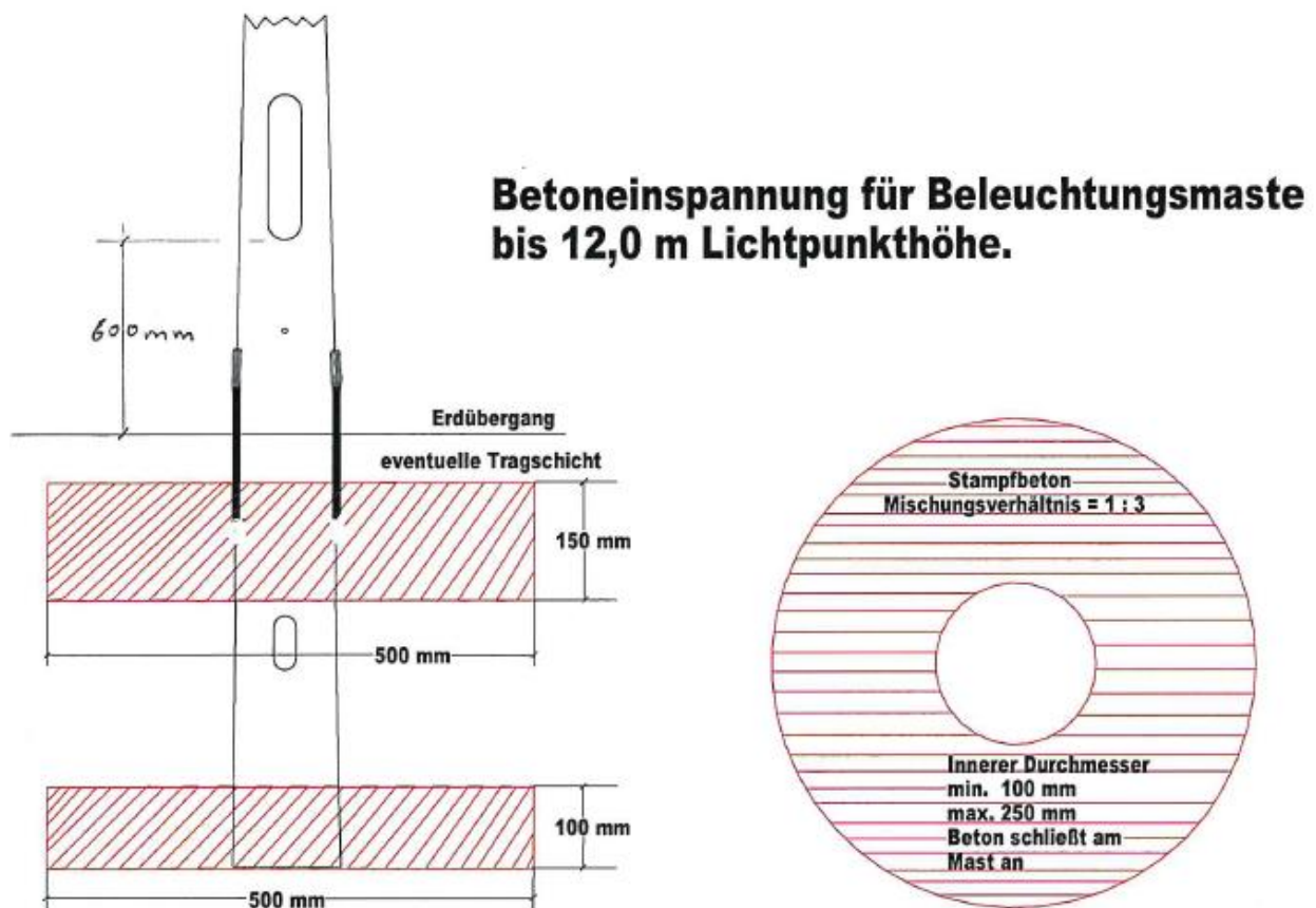
Abbildung 7 Betoneinspannung Straßenbeleuchtungsmast
