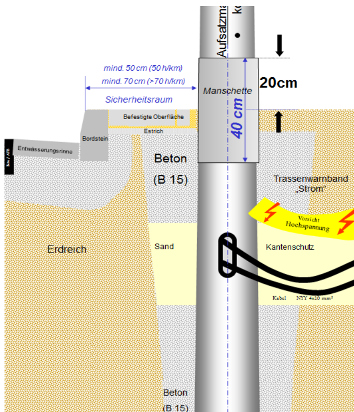
Abbildung 7 Betoneinspannung Straßenbeleuchtungsmast
