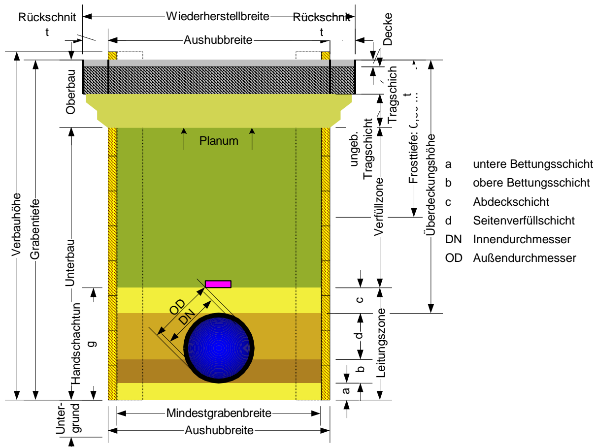
Abbildung 3 Standardgrabenprofil
